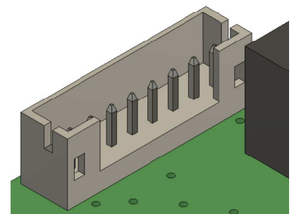
B8B-PH-K-S CN3 実装イメージ
