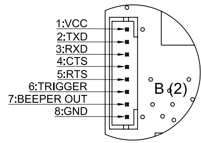
CN3 ピンアサイン
